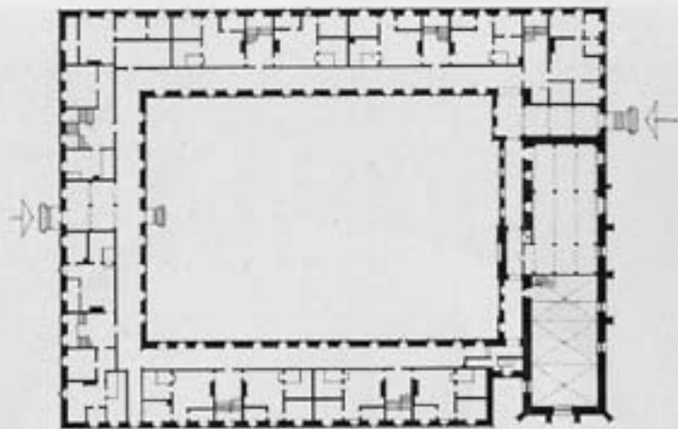
GRUNDRISS NÜTZE, DES KLOSTERGEBÄUDES
